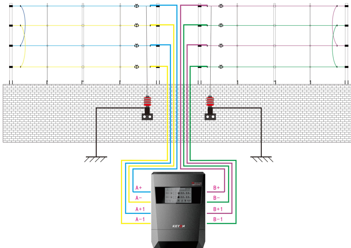
双防区四线制主机接线图
