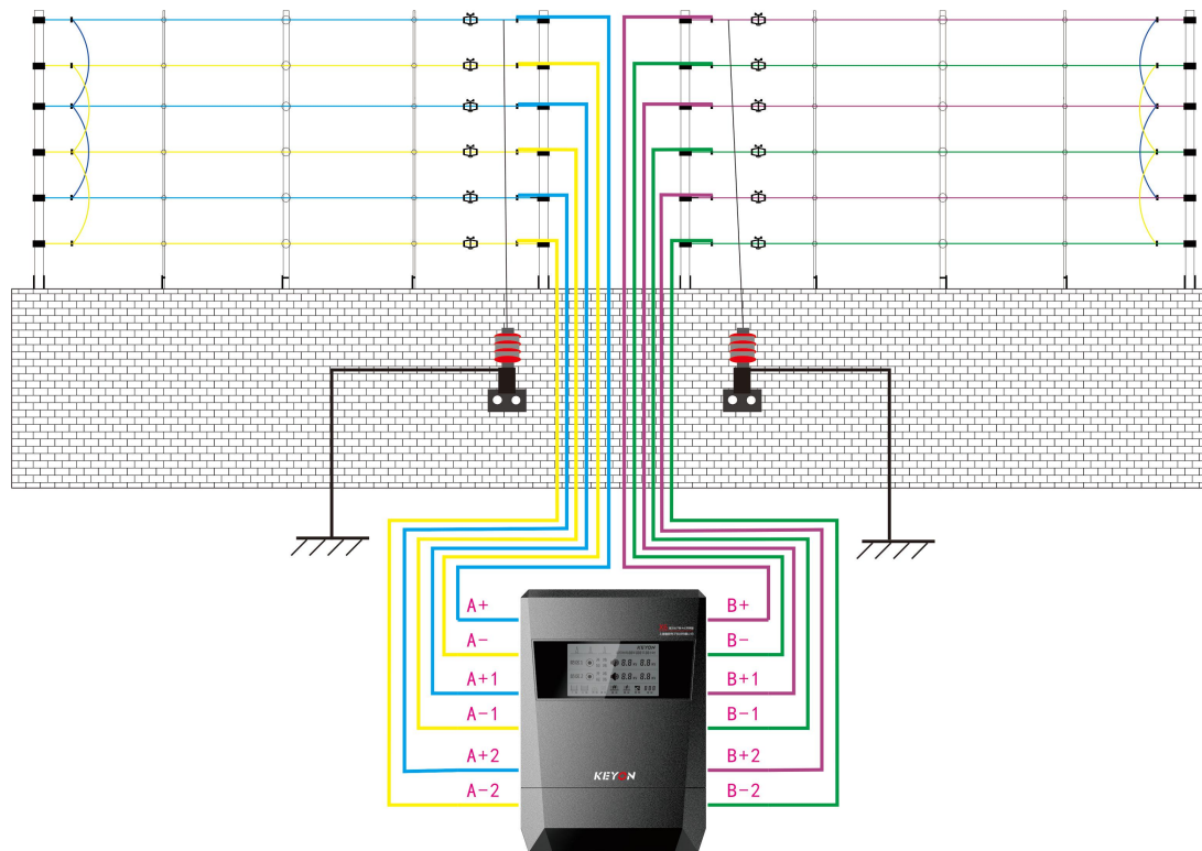
双防区六线制主机接线图
